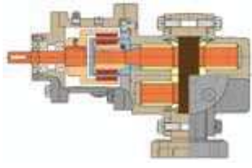
MC 構造図
