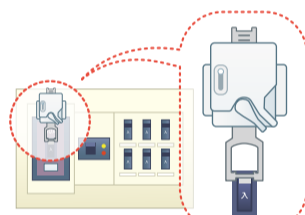
▲簡易型感震ブレーカーの例
