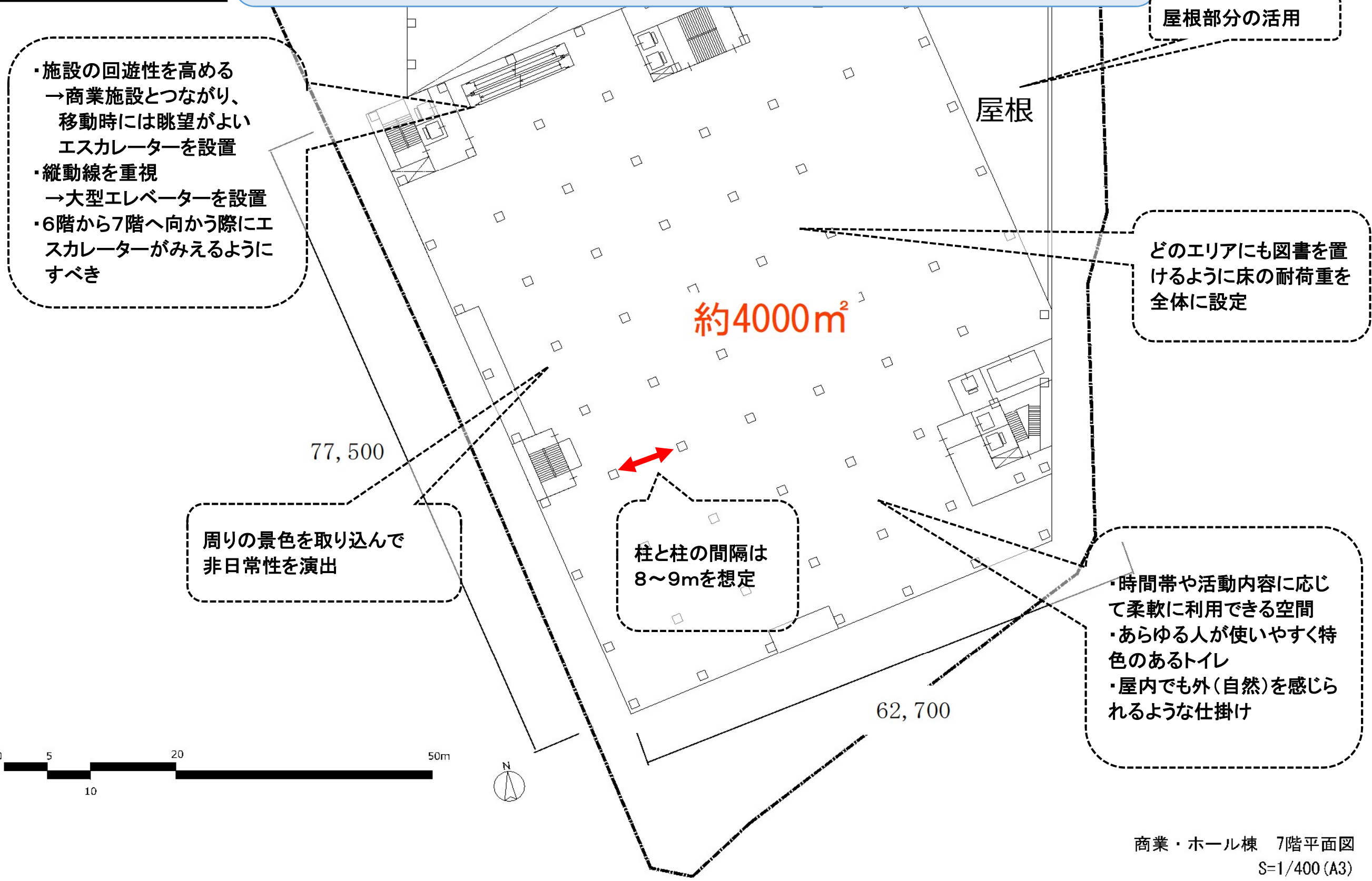
商業棟7階平面図
