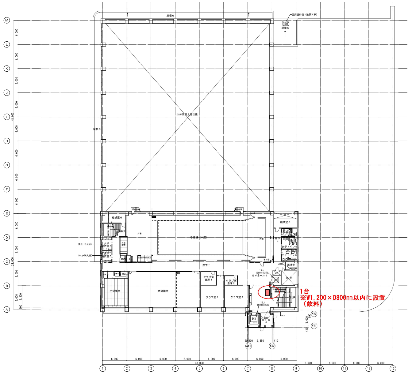
4階平面図【改修後】
