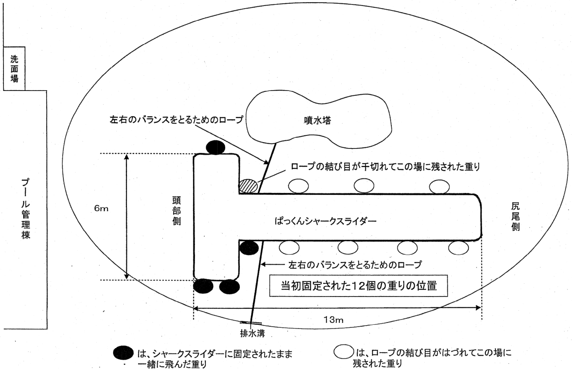
ぱっくんシャークスライダー重りの位置関係図
