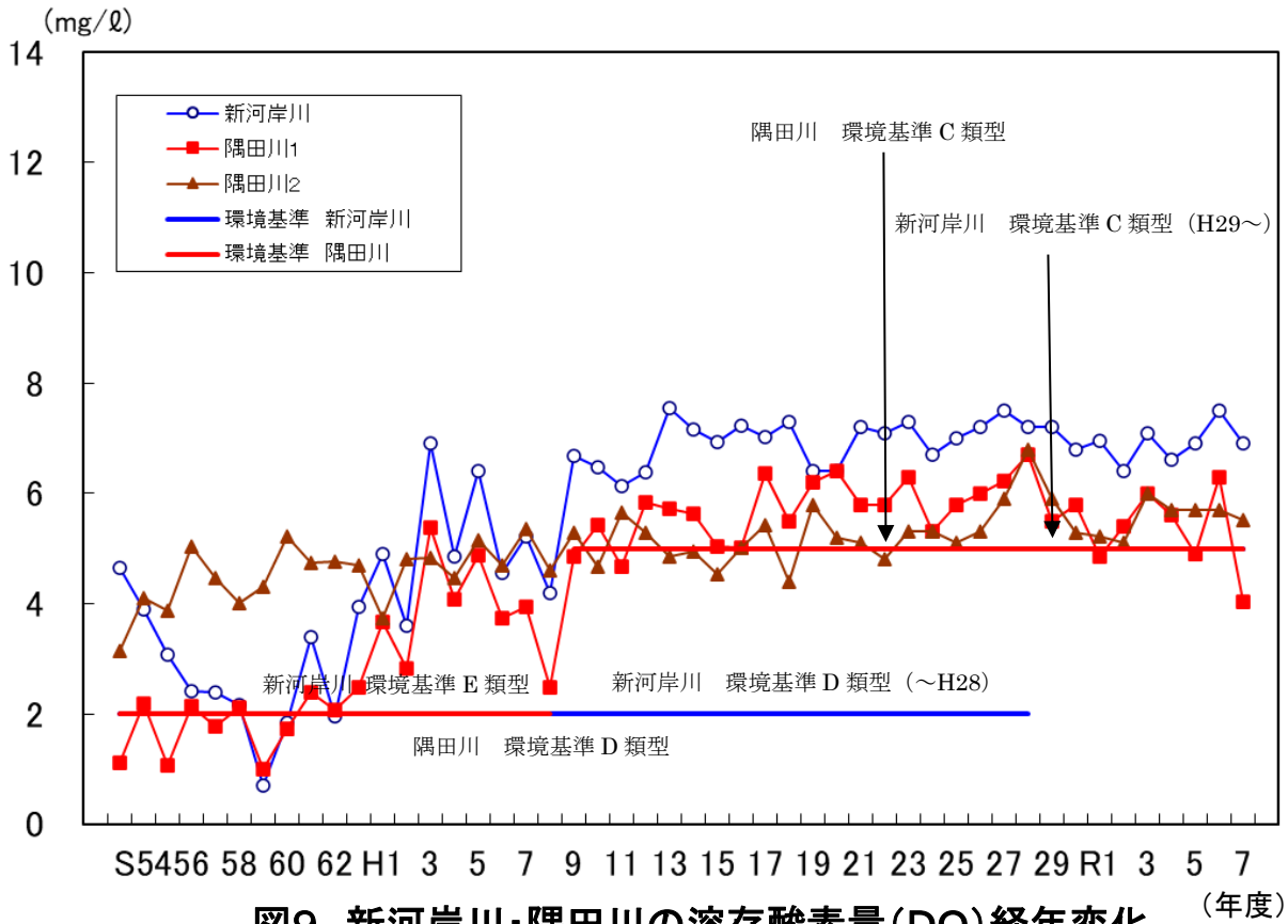
図9 新河岸川・隅田川の溶存酸素量(DO)経年変化
