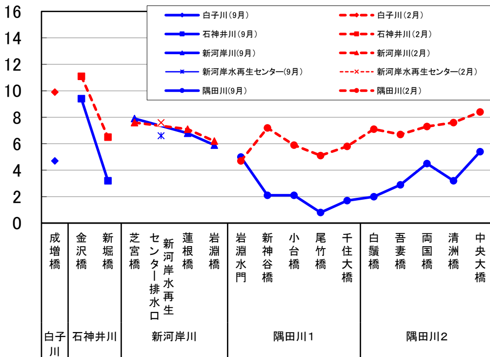
図1 溶存酸素量(DO)縦断変化
