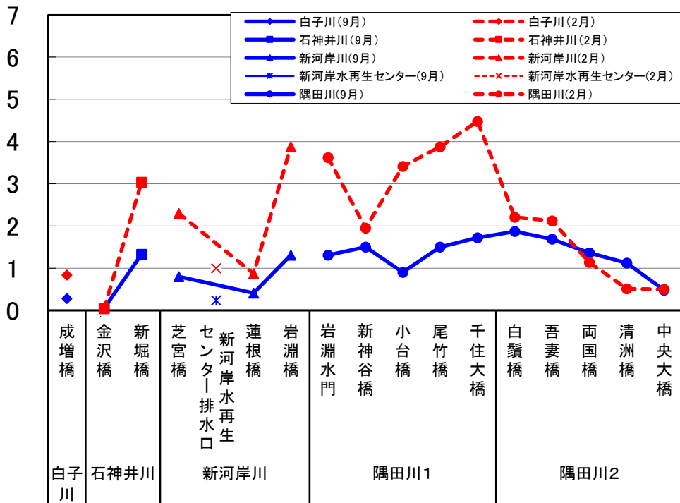
図8 アンモニア性窒素(NH4+-N)縦断変化
