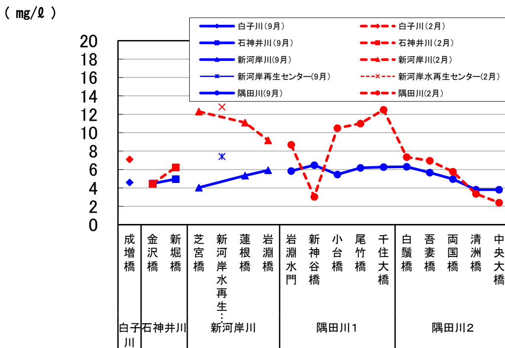
図6 全窒素(T-N)縦断変化
