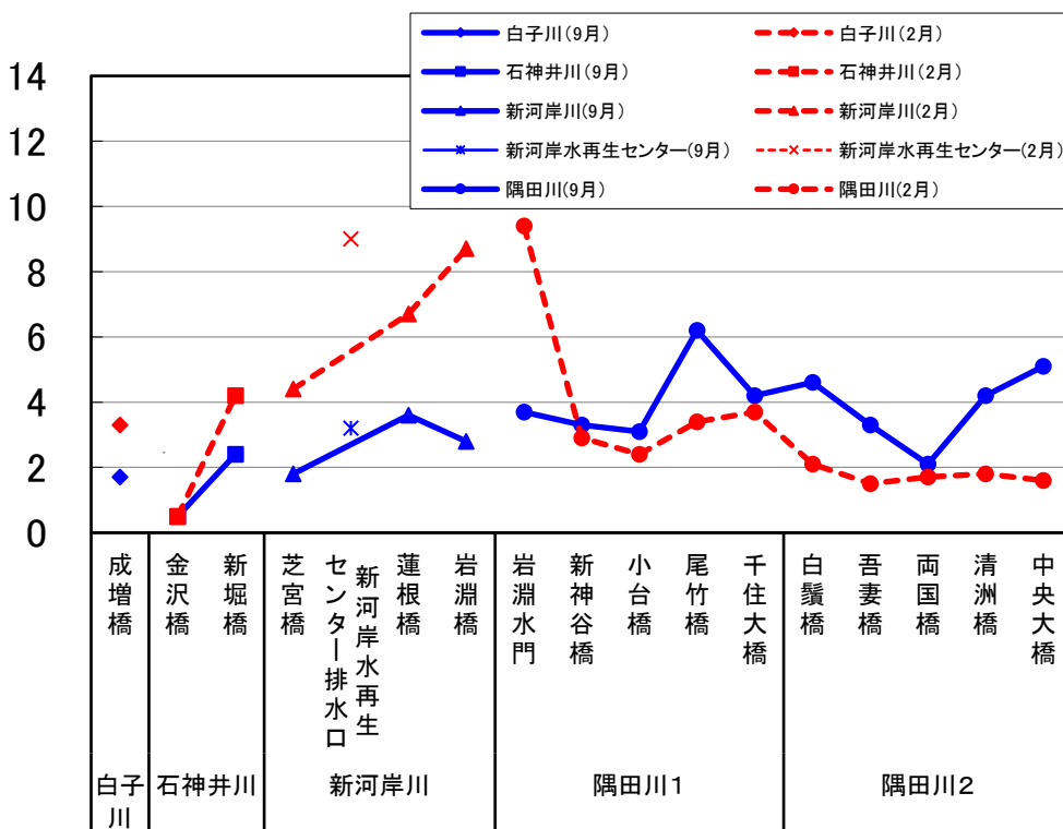
図2 生物化学的酸素要求量(BOD)縦断変化
