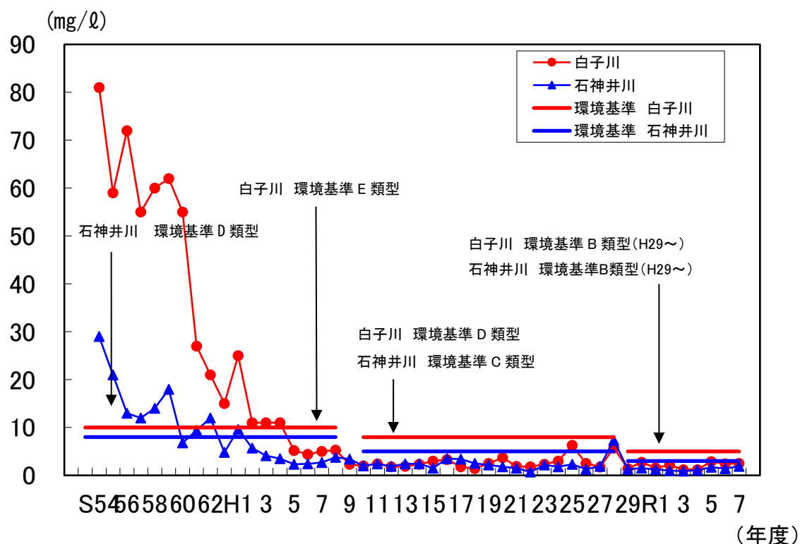
図12 白子川・石神井川の生物化学的酸素要求量(BOD)経年変化
