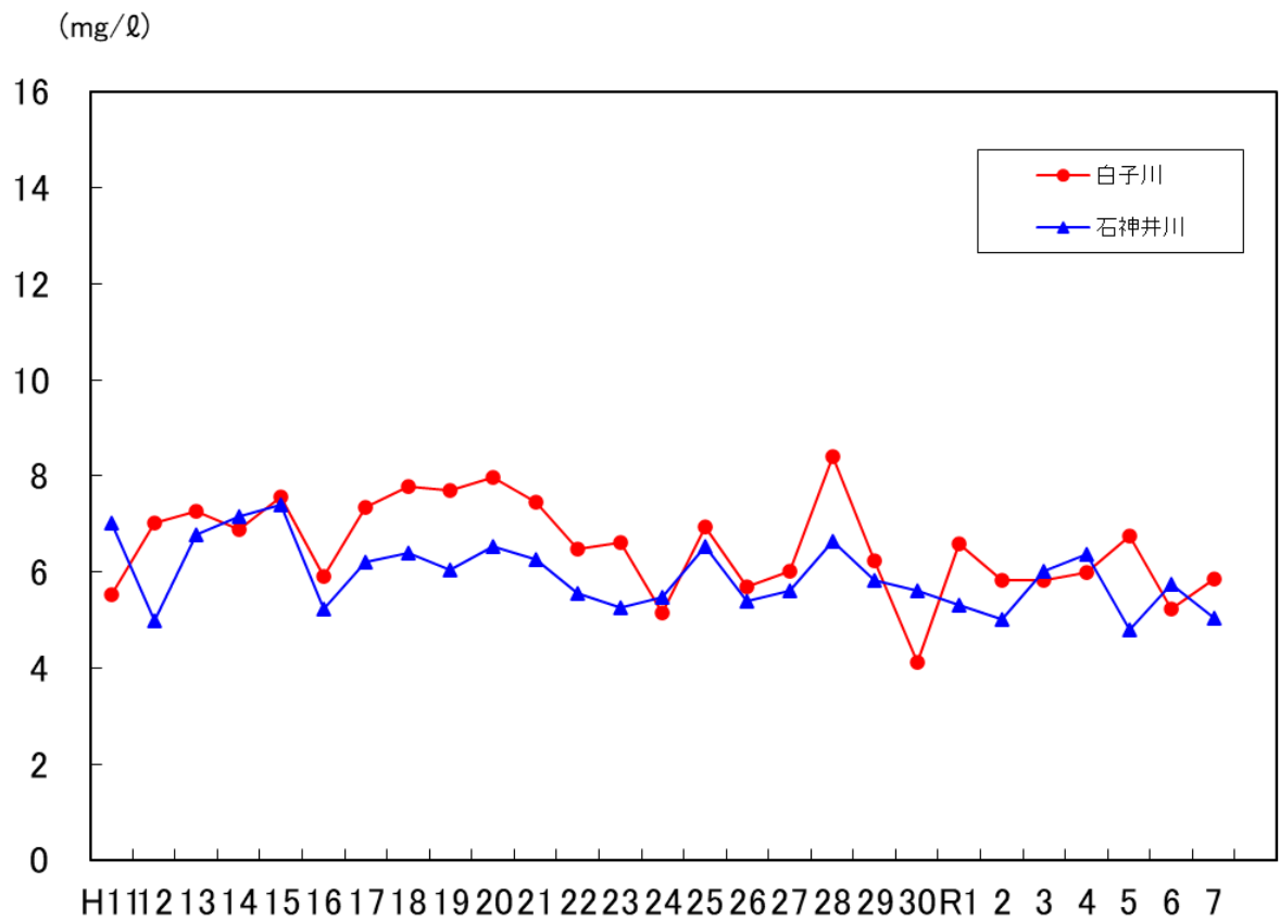
図15 白子川・石神井川の全窒素(T-N)経年変化 (年度)
