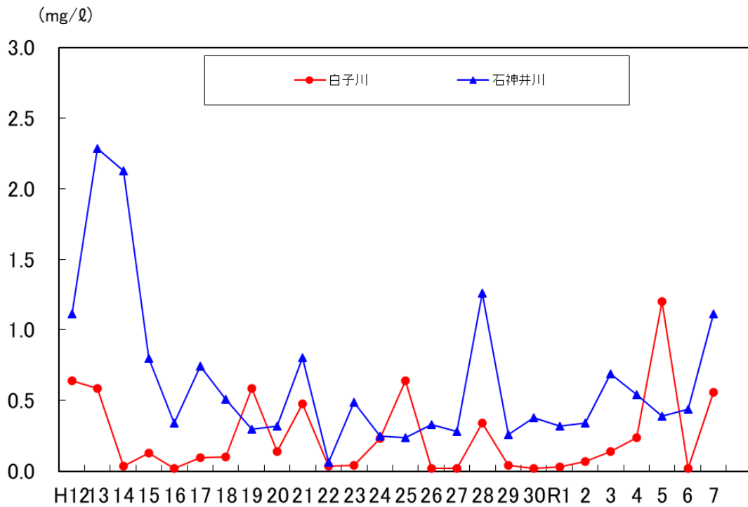
図 21 白子川・石神井川のアンモニア性窒素 (NH 4 + -N) 経年変化 (年度)
