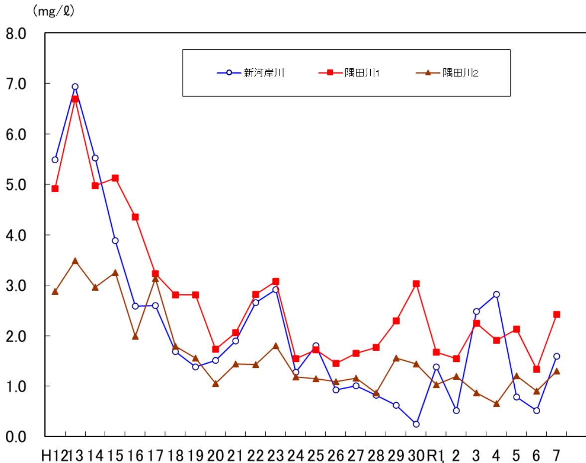
図 20 新河岸川・隅田川のアンモニア性窒素 (NH 4 + -N) 経年変化 (年度)
