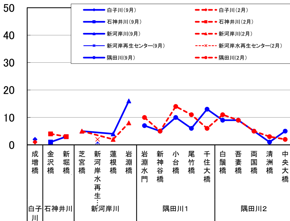
図4 浮遊物質(SS)の縦断変化
