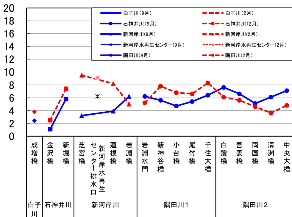
図3 化学的酸素要求量(COD)の縦断変化
