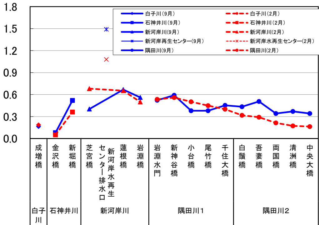
図7 全りん(T-P)縦断変化
